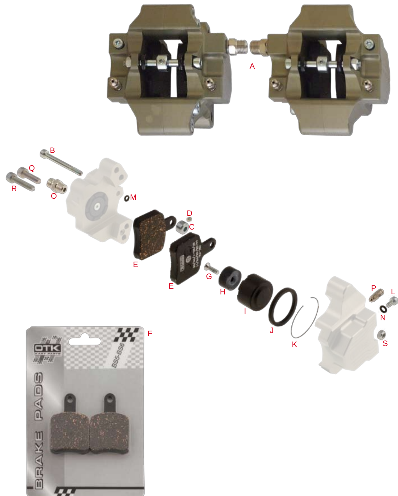
Tav. 34 PINZA FRENO ANTERIORE • FRONT BRAKE CALIPER BS5
