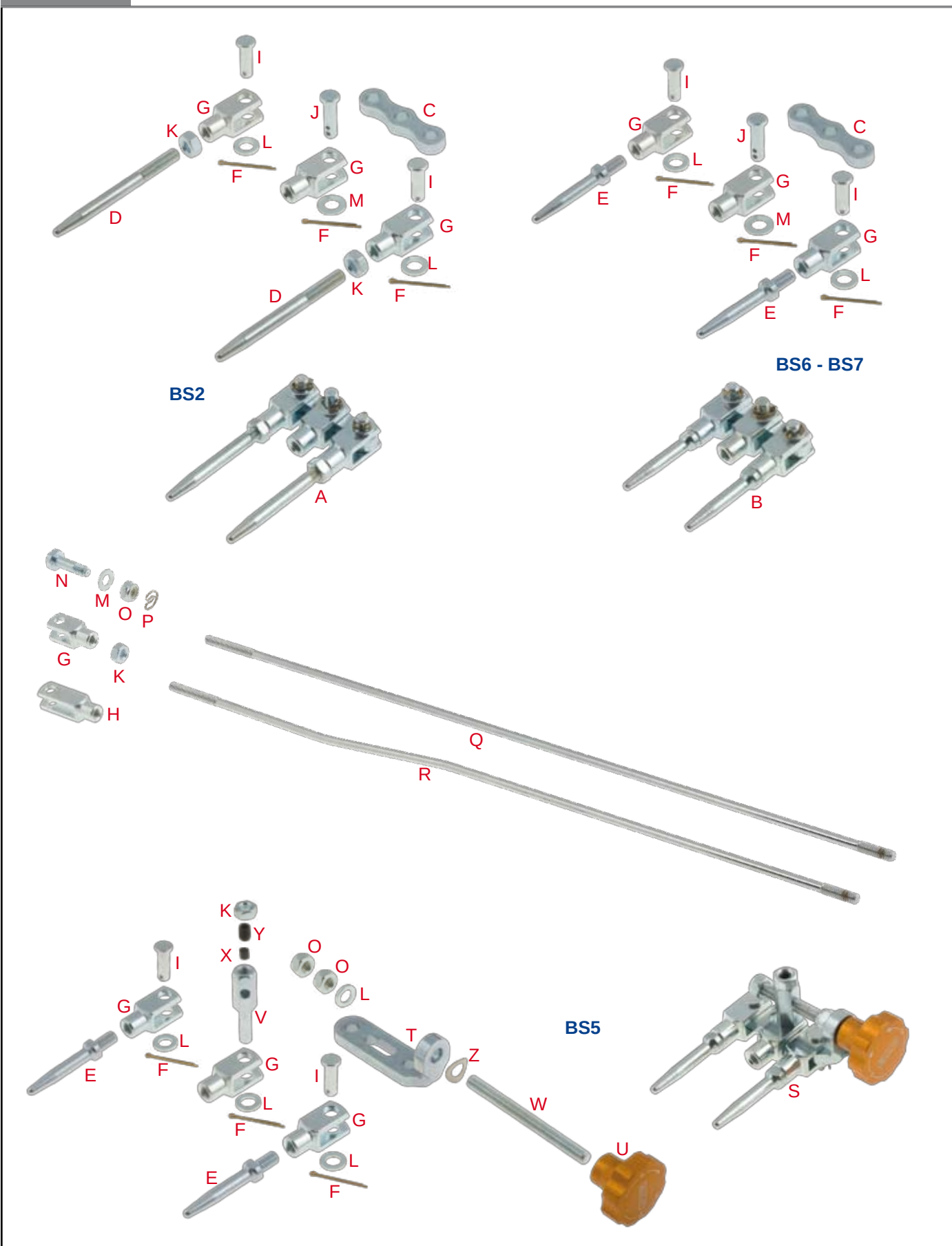
Tav. 37 GRUPPO PUNTALI E RIPARTITORE • PUSH RODS SYSTEMS AND LENGHTENING ARMS
