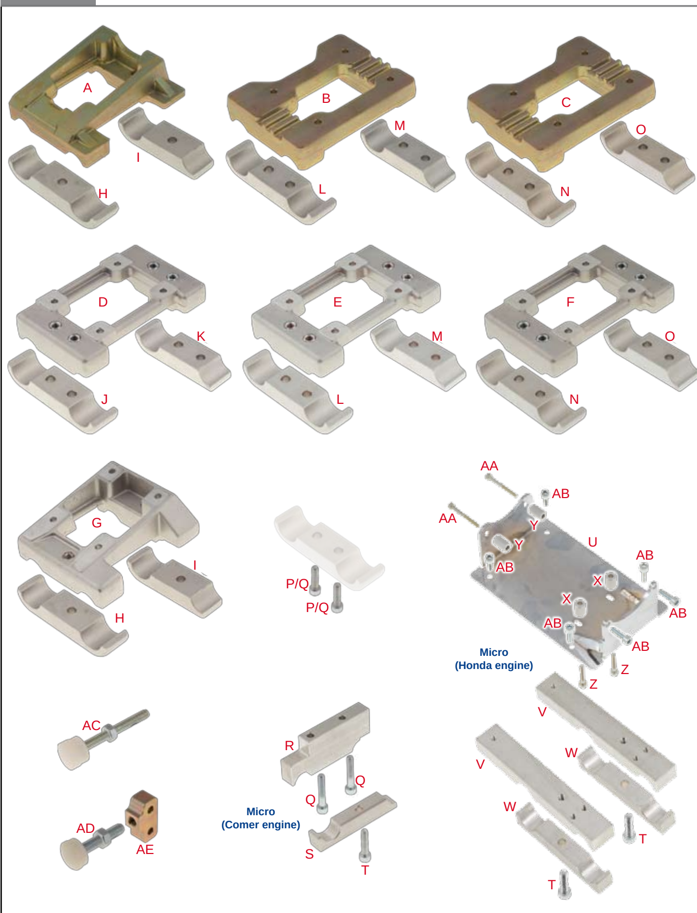
Tav. 13 PIASTRE MOTORE - ENGINE MOUNTS
