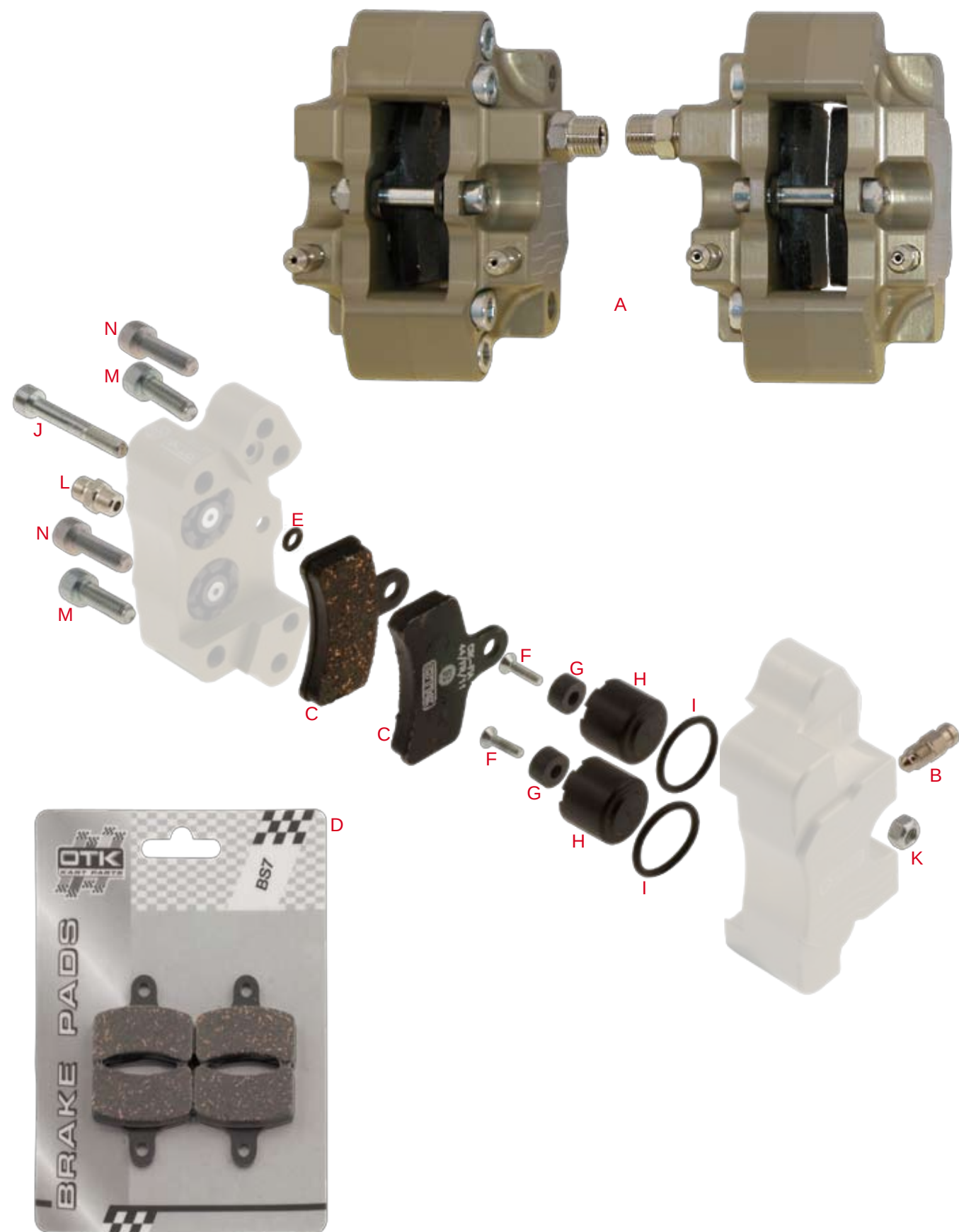
Tav. 35 PINZA FRENO ANTERIORE • FRONT BRAKE CALIPER BS7
